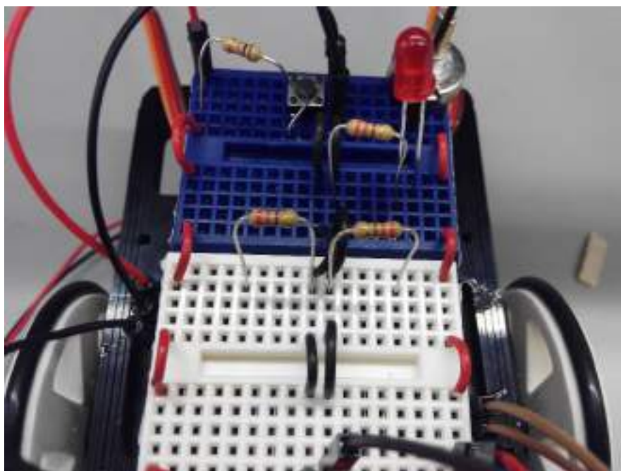
Poner las resistencias de 220\Omega
