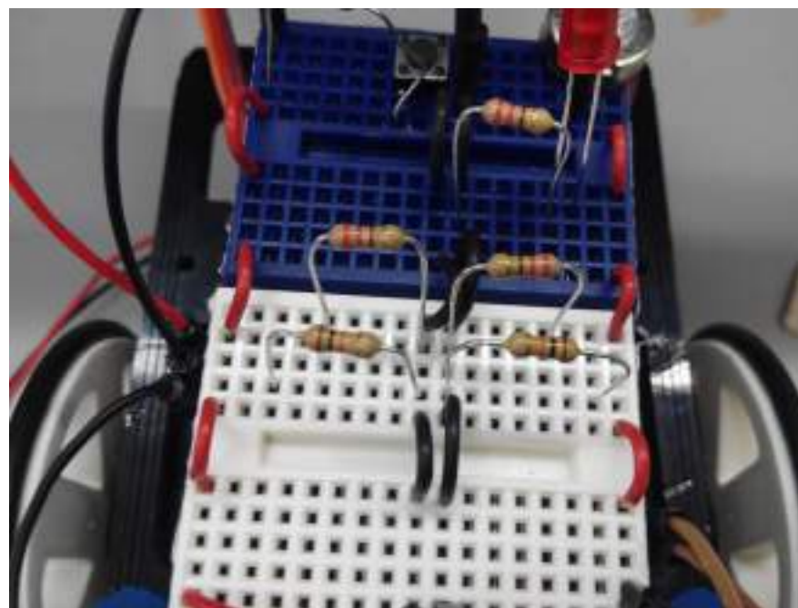
Poner las resistencias de 10k\Omega
